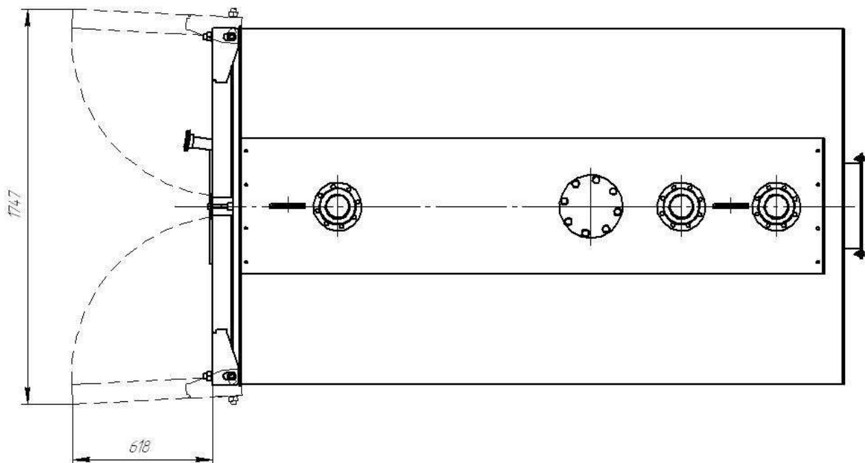
Рисунок 4. Схема открытия поворотных крышек.
