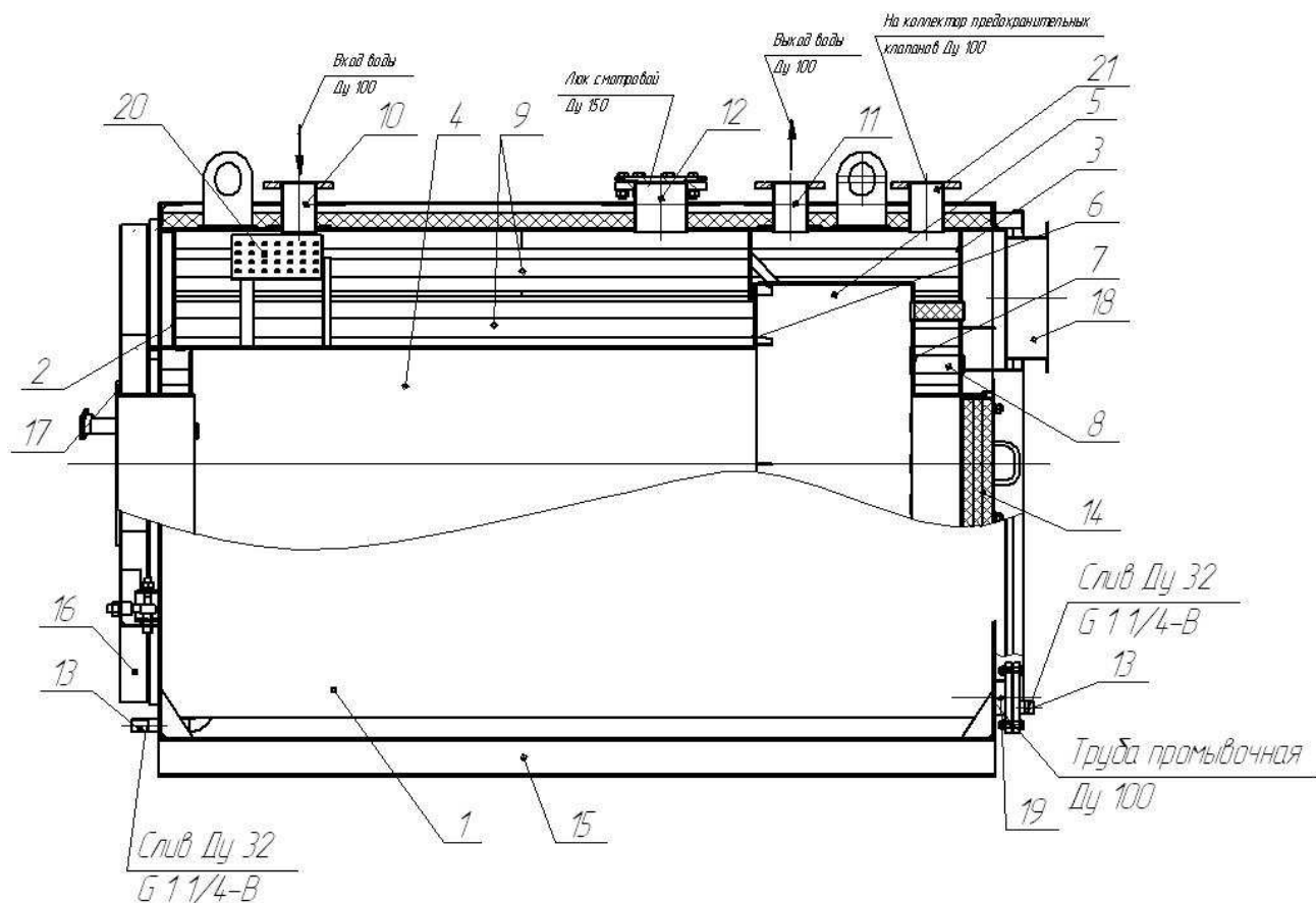
Рисунок 1. Схема котла
