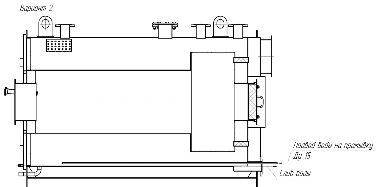
Рисунок 5. Варианты промывки котла.
