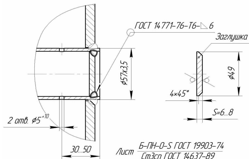
Рисунок 8. Установка заглушки.
