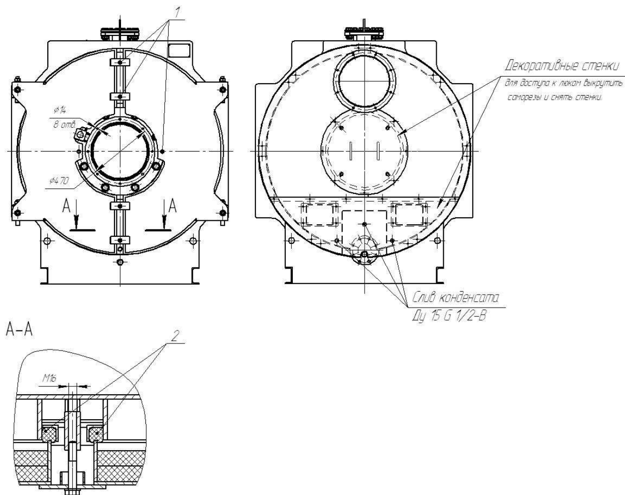
Рисунок 7. Фронтальная и задняя часть котла.
