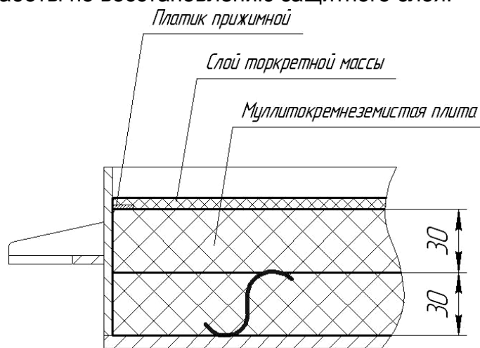
Рисунок 9. Разрез передней крышки.
