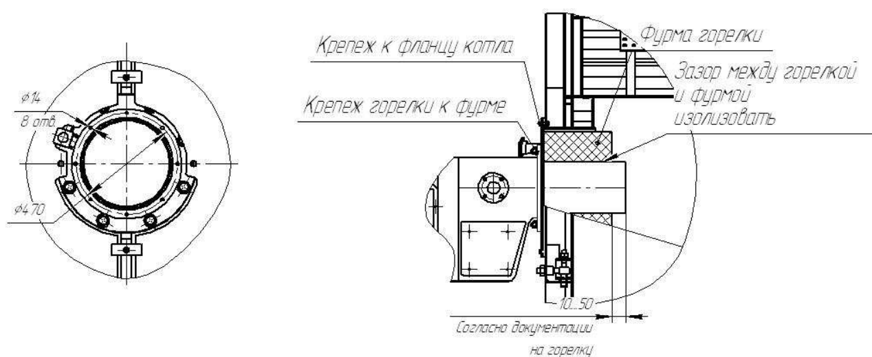
Рисунок 2. Фланец передний
