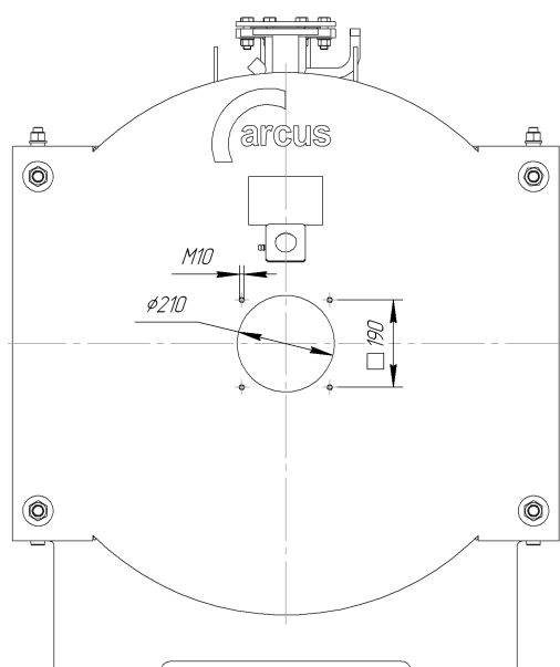
Рисунок 2. Крепление под фурму.
