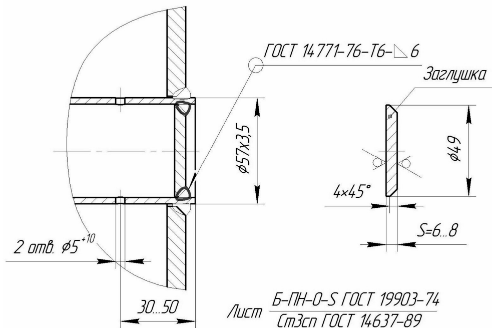
Рисунок 8. Установка заглушки.
