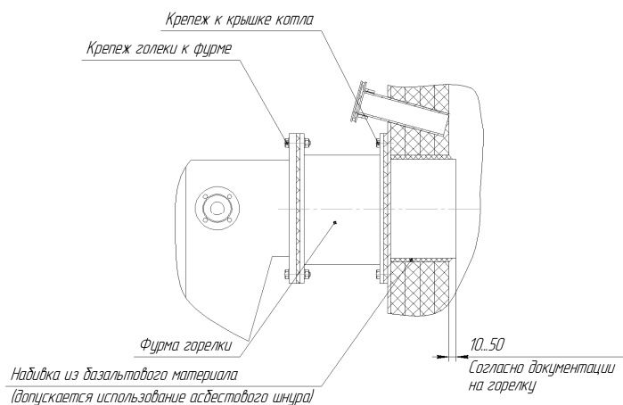
Рисунок 3. Крепление горелки.
