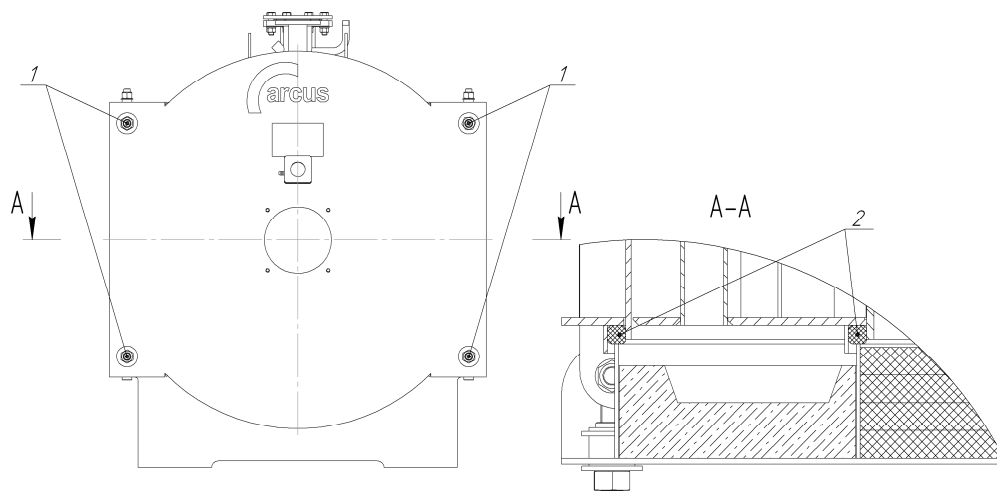
Рисунок 7. Передняя крышка.
