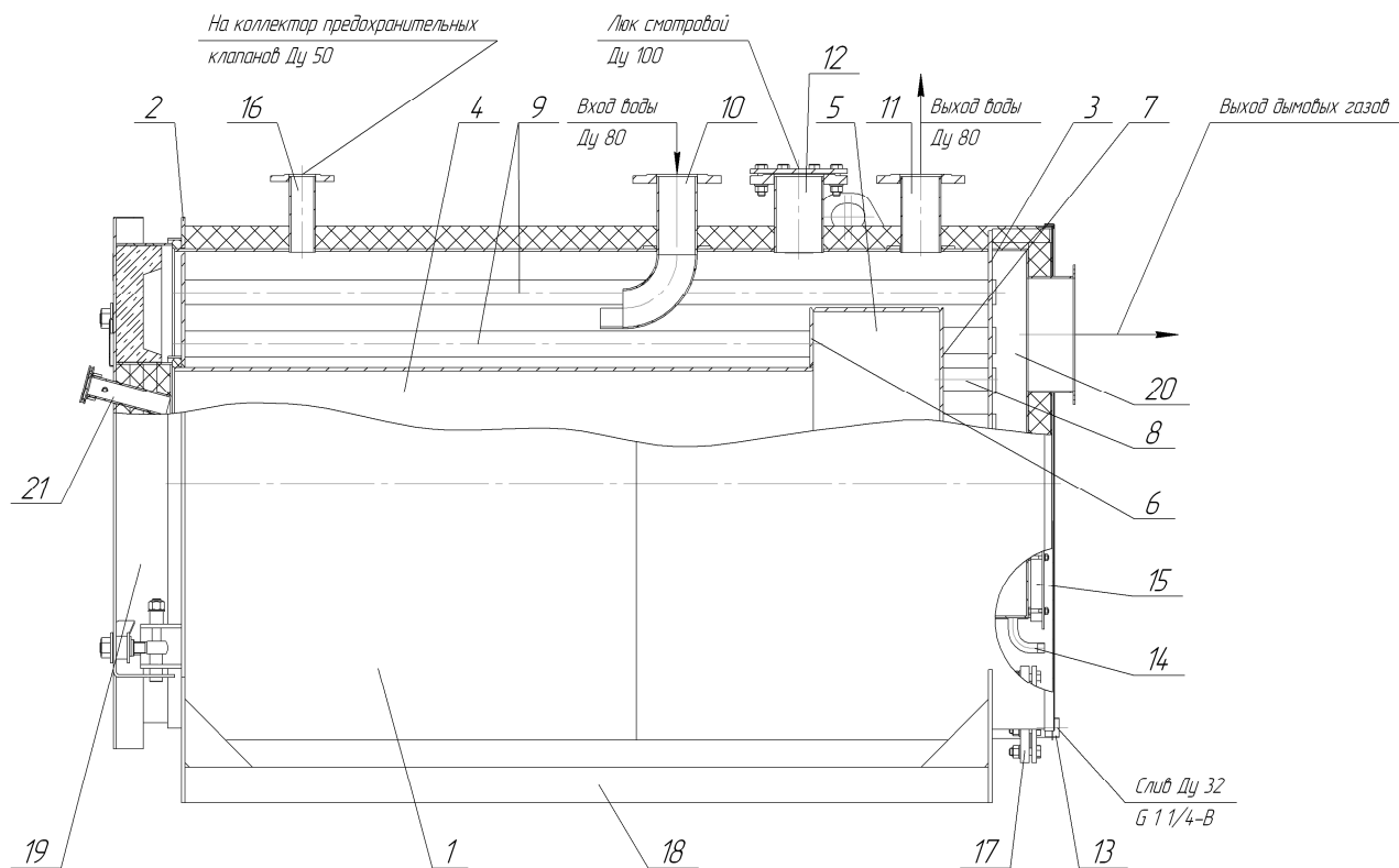
Рисунок 1. Схема котла
