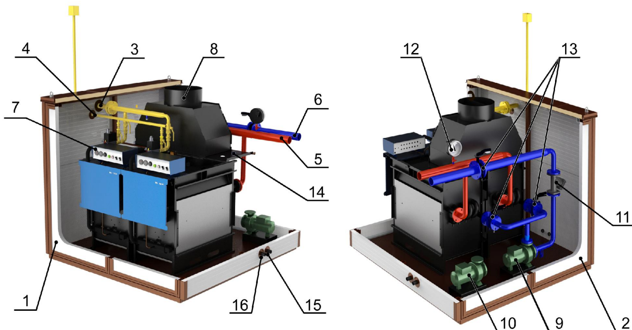
РИС.1 Внутренний вид сдвоенного котла наружного размещения.
