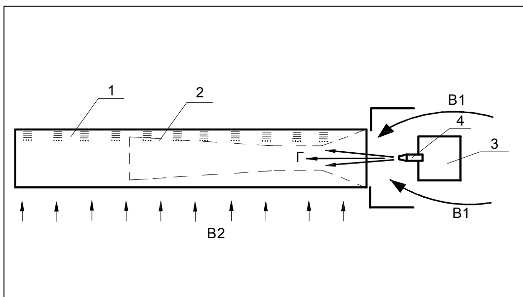
РИС.3 Устройство газовой горелки (вид сбоку)
