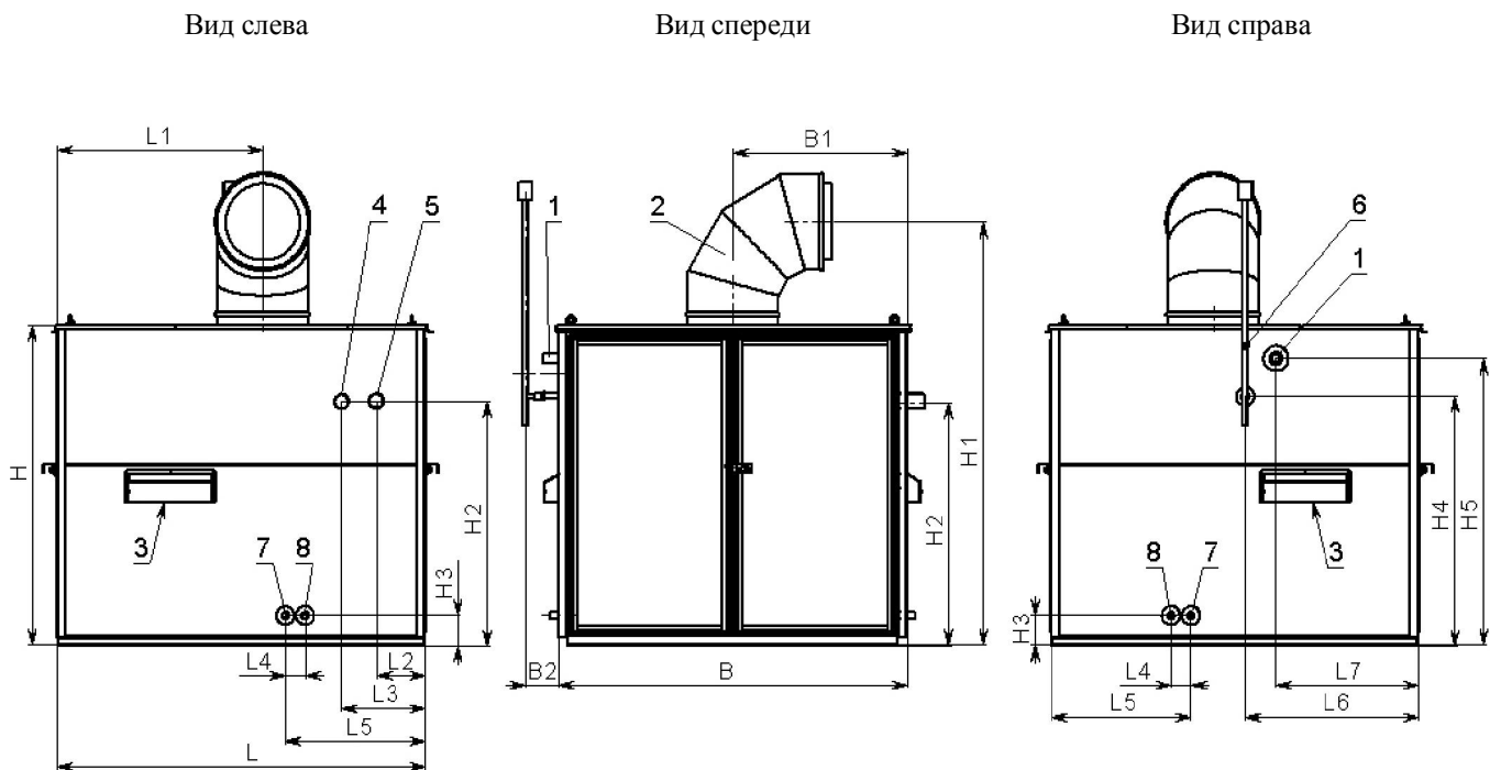
РИС. 4А Габаритно-присоединительные размеры для котлов RS-H80, 100, 150(КВа-0,12Гн), 150(КВа-0,16Гн), RS-H200.
