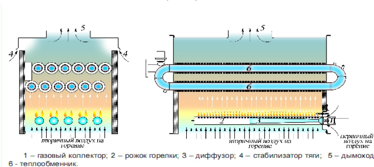
РИС.2 Принцип работы котла
