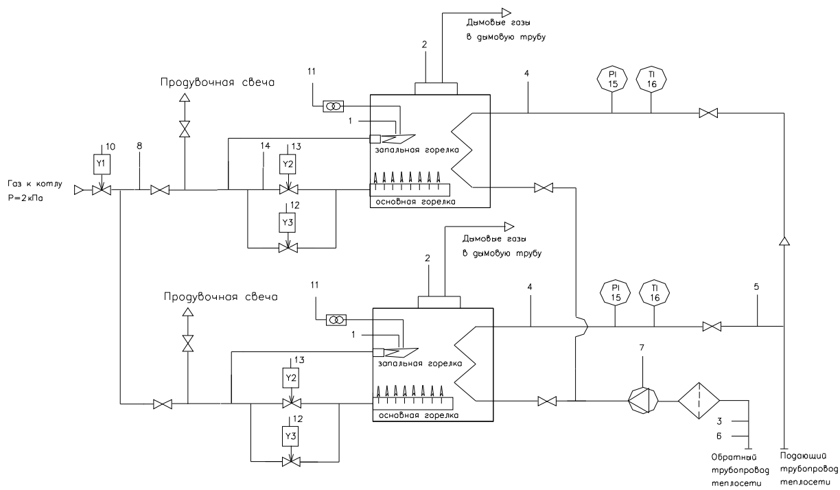
Функциональная схема автоматики сдвоенных котлов "RS-H 200 300, 400, 500, 600, 800"
