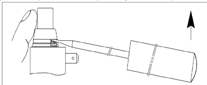
Рис. 18А Снятие колпачка с пилотного клапана
