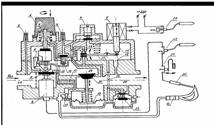
7.1 Устройство газовой автоматики «NOVA-820» на котле «RS-H80, 100, 150»
