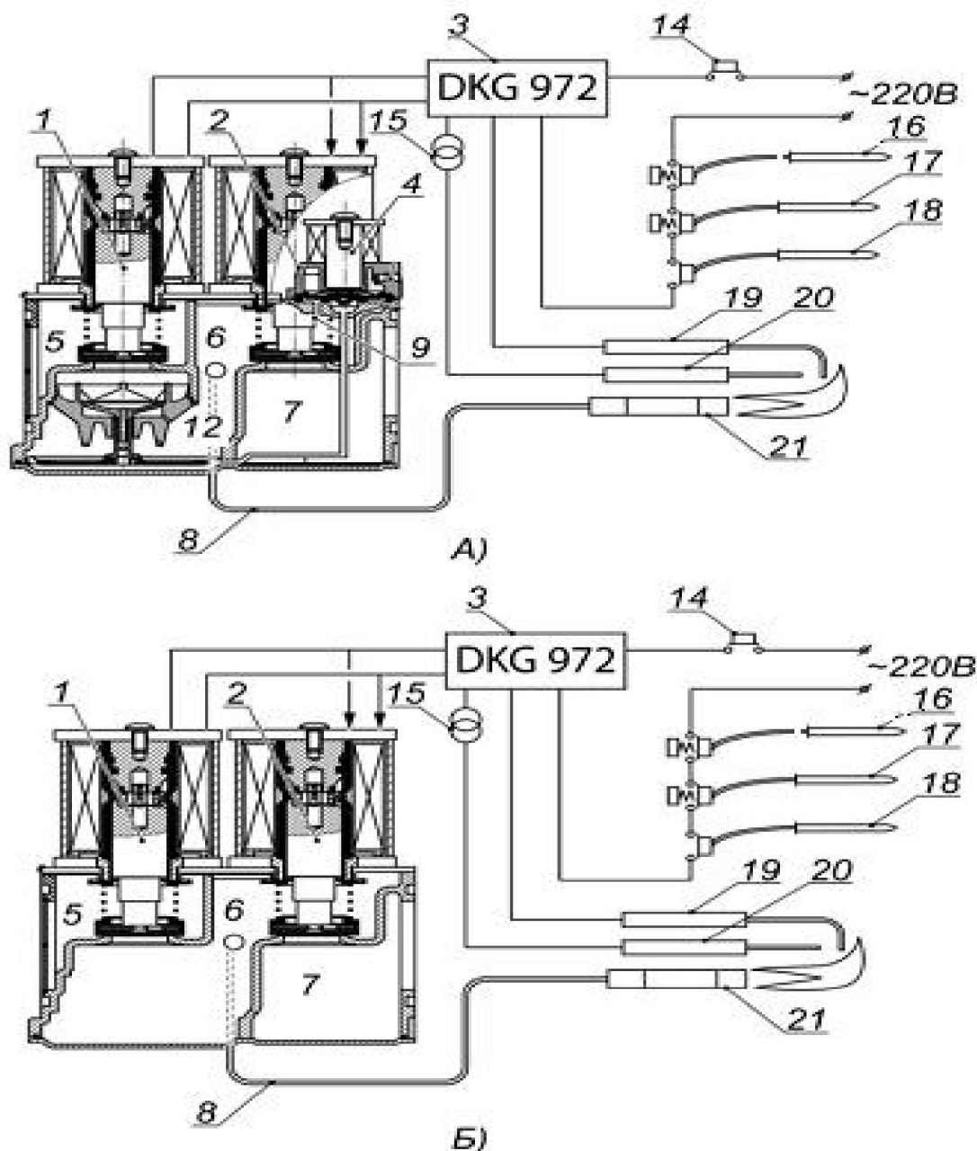
Рис.17. Устройство автоматики «HONEYWELL»: А) с клапаном VR 432, Б) с клапаном VQ 450M
