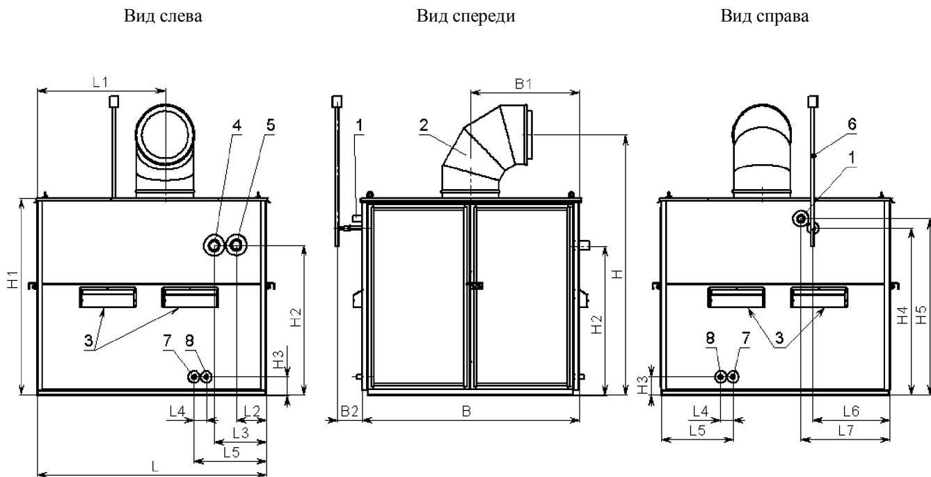
РИС. 4Б Габаритно-присоединительные размеры для котлов RS-H 300, 400, 500, 600:
