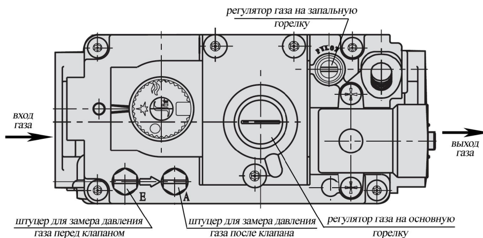
Рис. 6 Клапан NOVA 820, вид сверху
