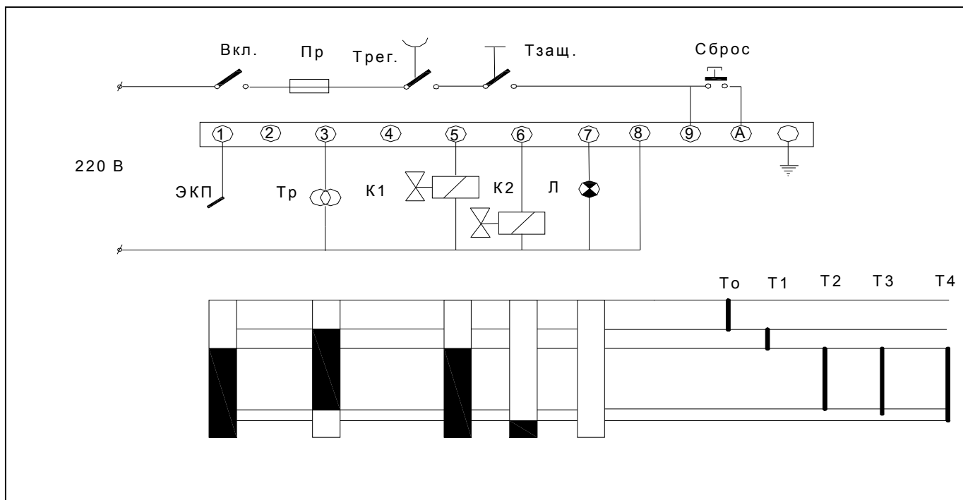
Рис. 20 Электрическая схема и временная диаграмма работы контроллера розжига
