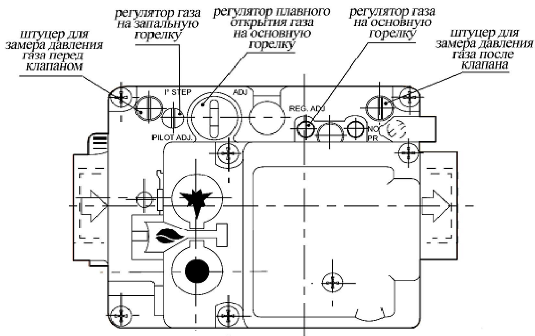
Рис. 9 Автоматика ELETROSIT-810 (вид сверху)
