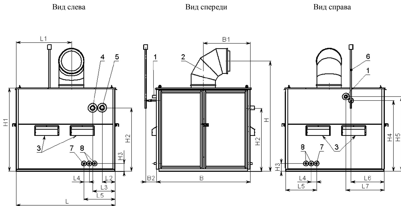
РИС. 4В Габаритно-присоединительные размеры для котла RS-H 800:
